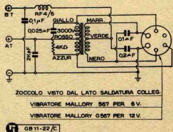
Vibratore
