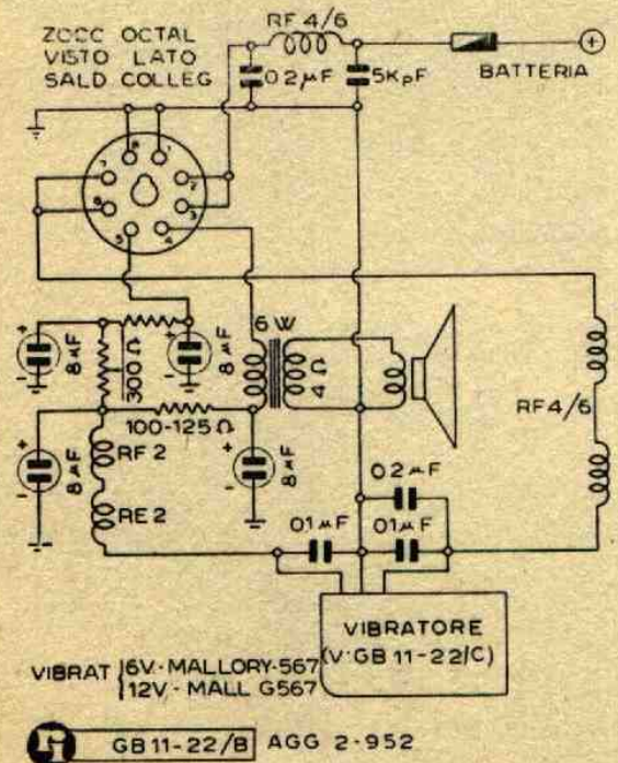
Alimentatore
