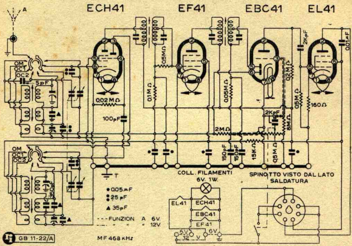
Lo schema elettrico del mod. "Saeita,": Sintonizzatore
